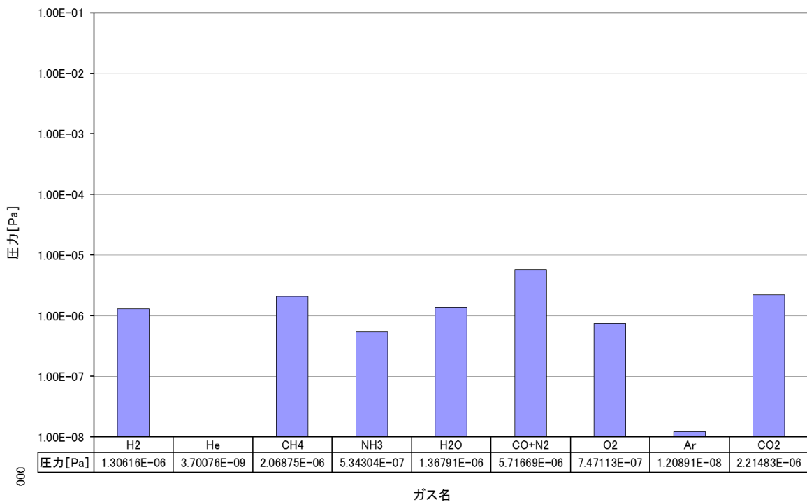
MVE-05H照明付きガス分析試験 分圧グラフ(本体 48時間経過)
