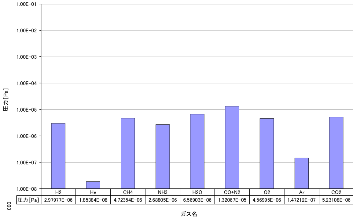
MVE-05H照明付きガス分析試験 分圧グラフ(本体 24時間経過)
